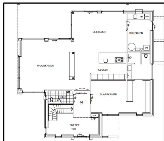
Afbeelding 4 & 5. Bouwtekeningen woning Warmoltsstrjitte 130 te Harkema
